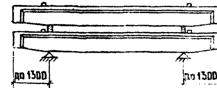
СХЕМА ОПИРАНИЯ БАЛОК ПРИ ПЕРЕВОЗКЕ И ХРАНЕНИИ
